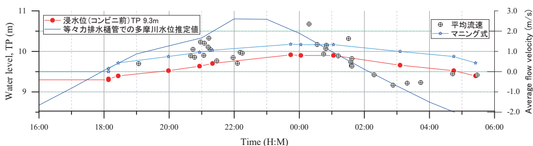
図5 浸水位と平均速度の時間変化
