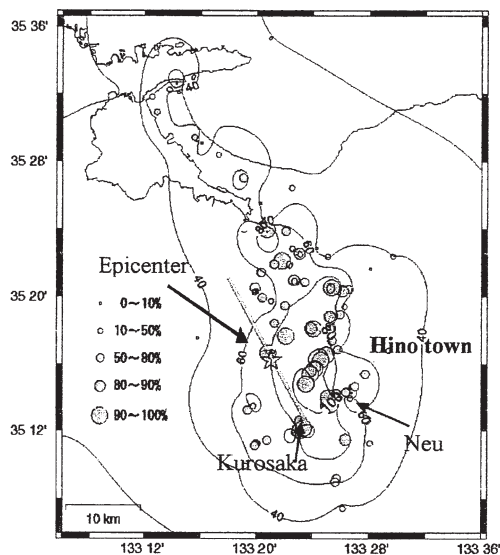
図 1 2000 年鳥取県西部地震震央と日野町の位置 6)
